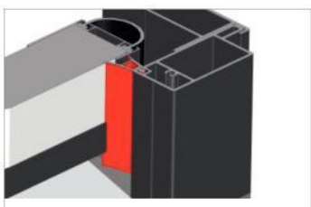
Joint tubulaire à lèvre EPDM côté fermeture
