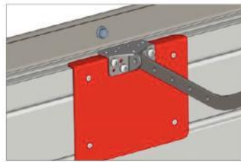
Plaque renfort pour liaison du bras moteur
