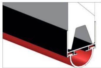
Joint à bulle EPDM sur panneau bas
