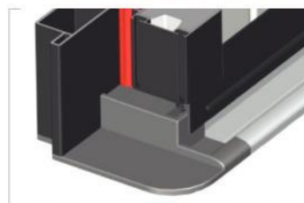
Joint d'étanchéité tubulaire EPDM côté ouverture
