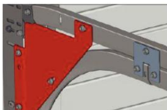
Plaque renfort sur courbes
