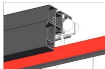
Joint d'étanchéité EPDM sur linteau
