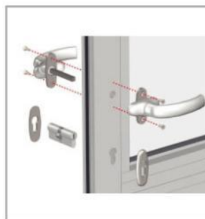
Poignée avec rosaces et canon de sécurité
