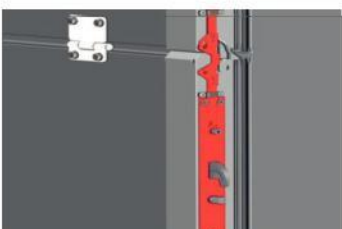
Serrure à crochets haute et basse
